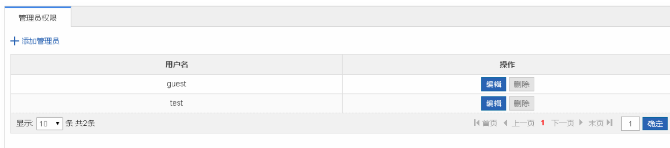
图 1-51 管理员权限
